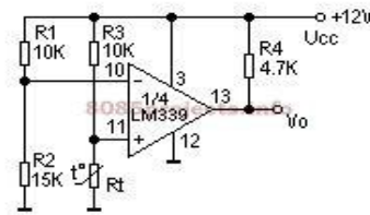
FIG: 2 Zero Crossing Detector Module
