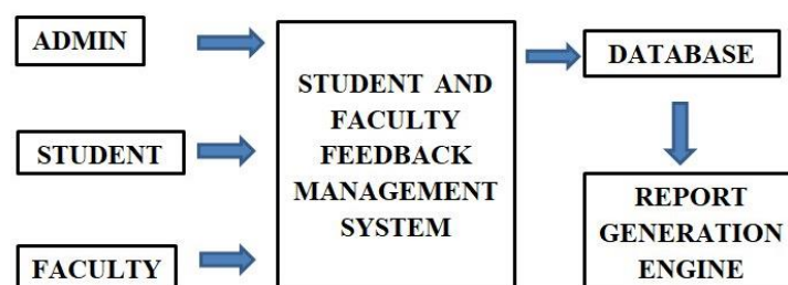
Fig. IV. a. Implementation
